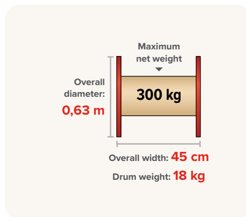
DRUM Ø 630
